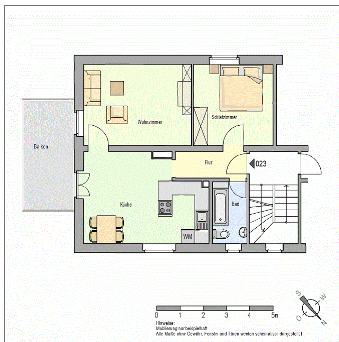
- Grundriss
