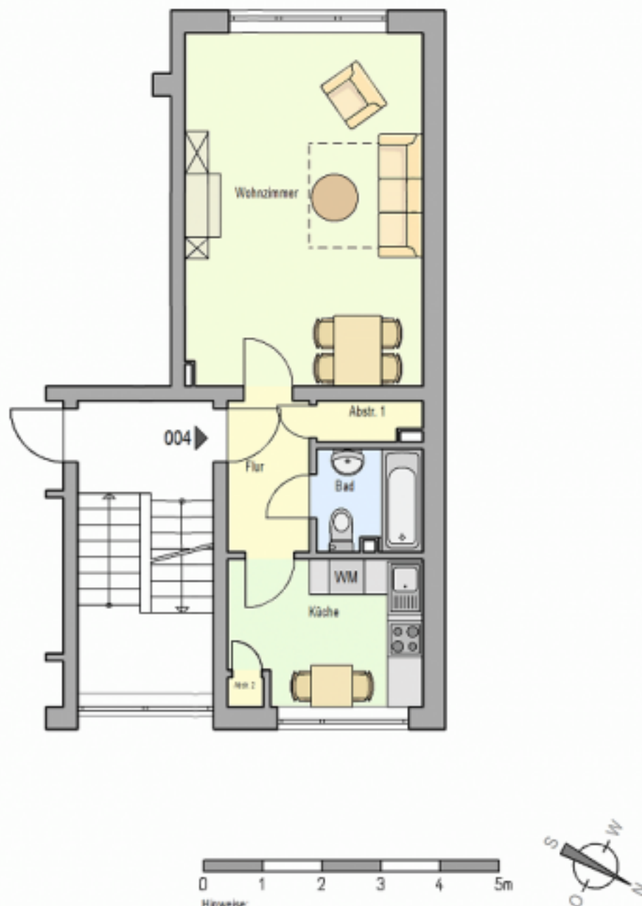
- Grundriss
